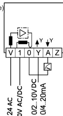
Схема подключения артикул № 115 80 20
