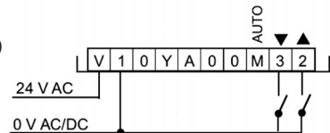
Схема подключения артикул № 115 80 20
