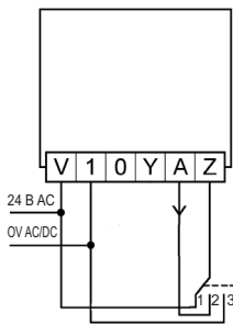
Схема подключения артикул № 115 80 21 / 22
